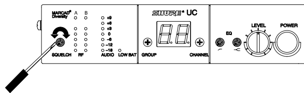
EINSTELLEN DER RAUSCHSPERRENWERTE FÜR DEN EMPFÄNGER UC4
