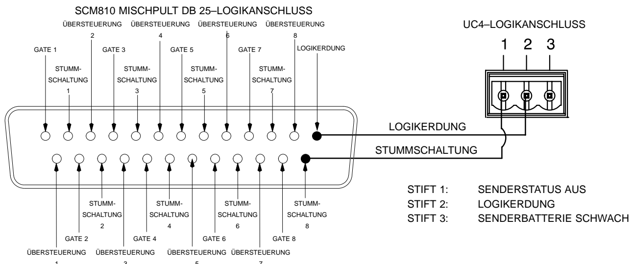
TYPISCHE UC4-ANSCHLÜSSE AM LOGIKANSCHLUSS DES MISCHPULTS SCM810
